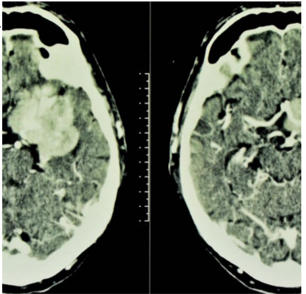
La ricerca conferma il coinvolgimento di Skt nei processi cognitivi
